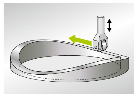
Accionamento da bomba de vácuo por um excêntrico (esquematicamente)
