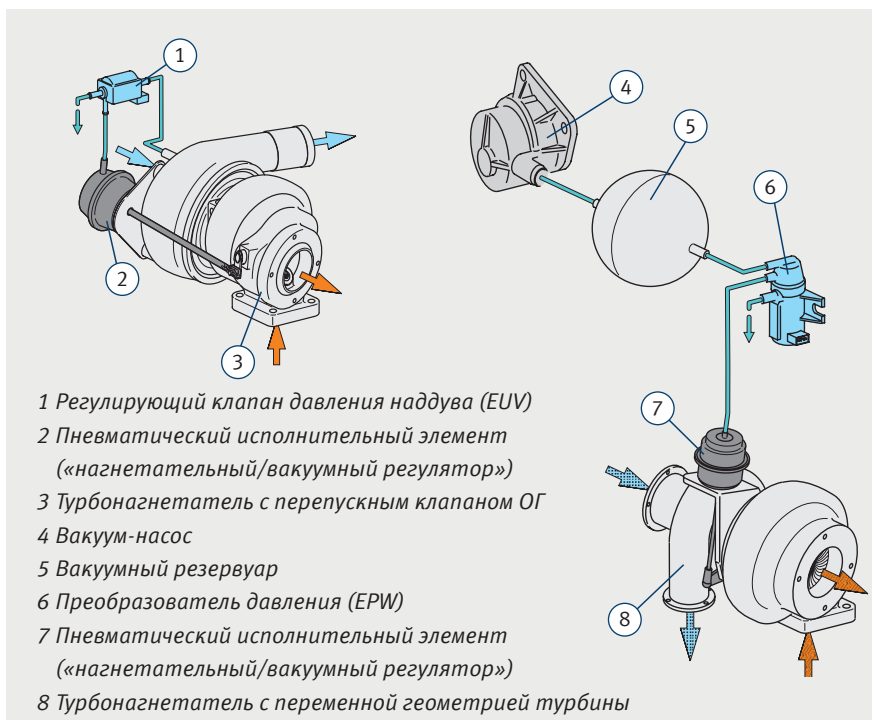
Пример: турбонагнетатель с переменной геометрией турбины и EPW (выделены красным цветом) в Audi A4 TDI
