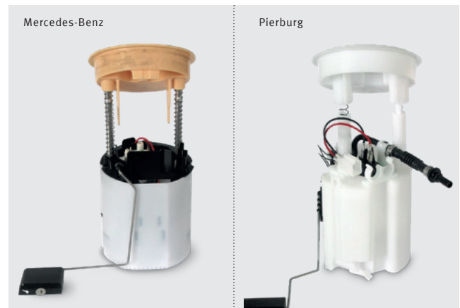
Fig. 1 : comparaison des modules d'alimentation en carburant
