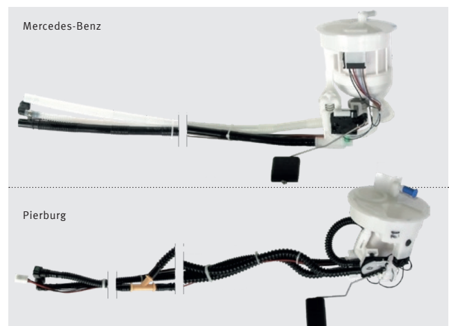
Fig. 2 : comparaison des unités d'indicateur de niveau
