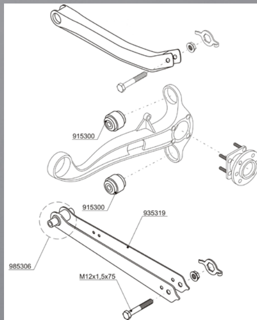
Bild 1: Achsstrebe Opel Vectra Hinterachse
