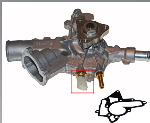
Bild 2: 65384 (mit Temperatursensor)
