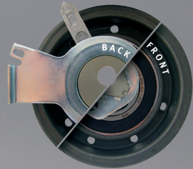
Bild 2: 55443 (neue Ausführung)
