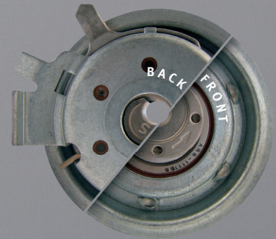
Bild 1: 55443 (bisherige Ausführung)
