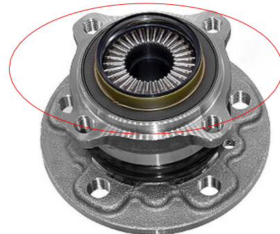
Alte Ausführung MIT Zentrierkappe Neue Ausführung OHNE Zentrierkappe
