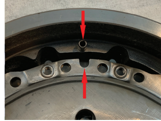
Şekil 2: Doğru Montaj
