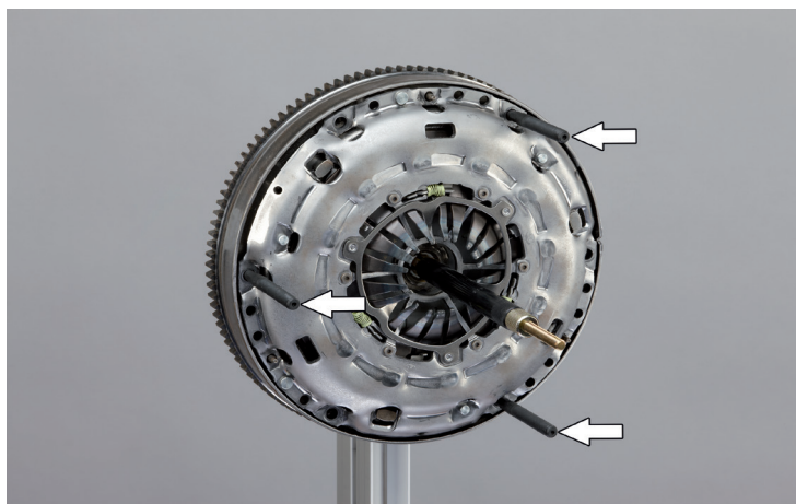
Bild 2: Stehbolzen zur Aufnahme des Spindelträgers
