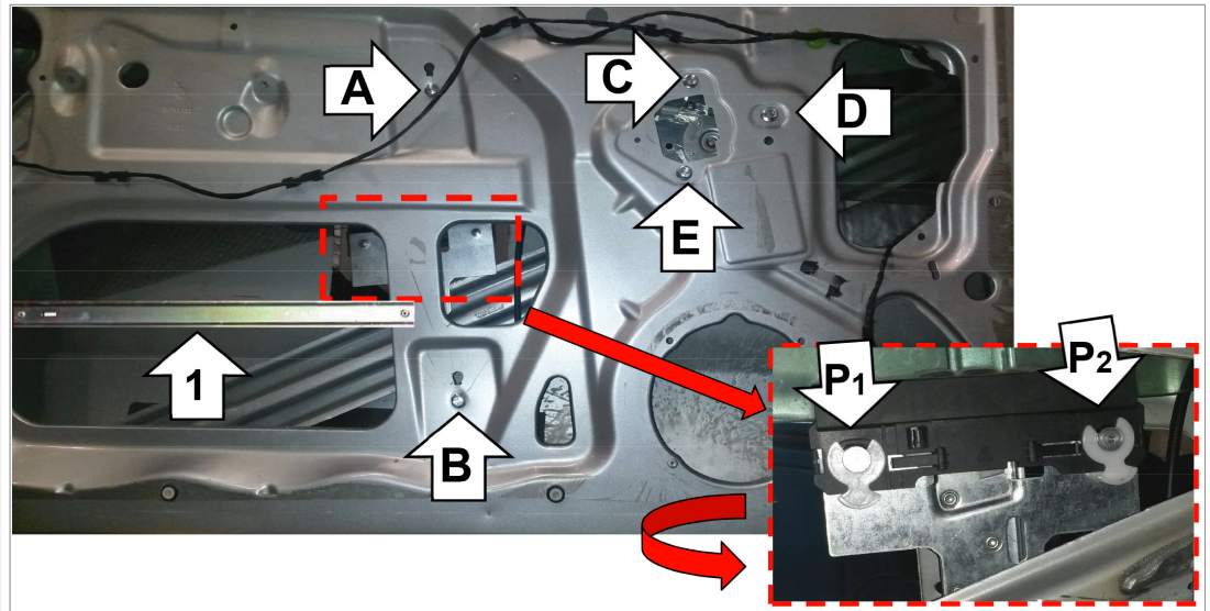
POWER WINDOW LEFT ALZACRISTALLI ELETTRICO SX
