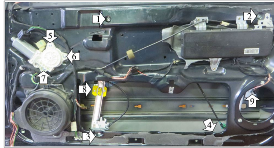
A POWER WINDOW RIGHT ALZACRISTALLI ELETTRICO DX
