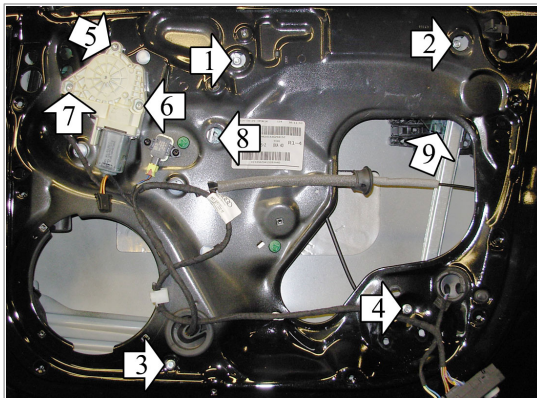
A POWER WINDOW RIGHT ALZACRISTALLI ELETTRICO DX
