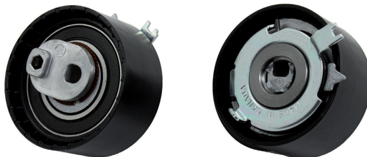
Bild 1: INA-Spannrolle 531 0409 30
