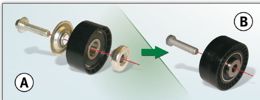
Umlenkrolle 532 0433 10, bisherige Ausführung (A) und neue Ausführung (B)
