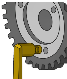
Přípravek pro zajištění setrvačnicku
