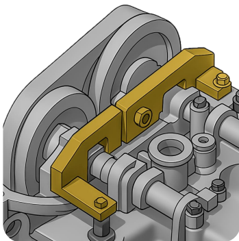
Přípravky pro nastavení váčkového hřídele
