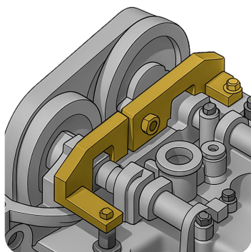
Přípravky pro nastavení vačkového hřídele
