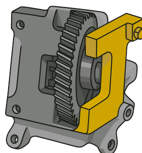
Přípravek na nastavení vačkové hřídele
