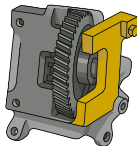
Přípravek na nastavení váčkové hřídele
