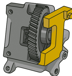
Přípravek na nastavení vačkové hřídele
