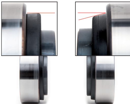
Bild 1: Das Design des Staubschutzdeckels wurde geändert
