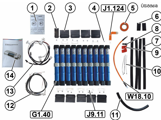
Abbildung 1 HV- Batterie Reparatursatz Kit - Lieferumfang
