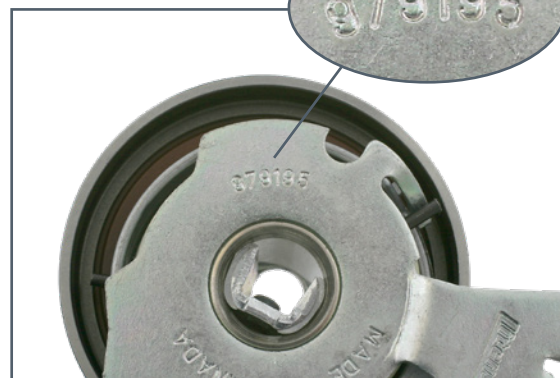
febi 10297 / SWAG 40 03 0028
