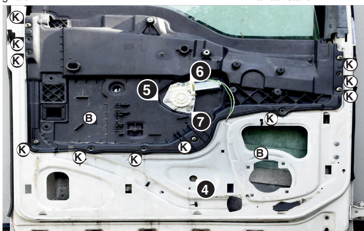
oem window regulator - lève-vitre original - Fensterheber von oem - eleva-lunas original - levantator de vidro original - Γρύλος γνήσιος - alzacristallo originale
