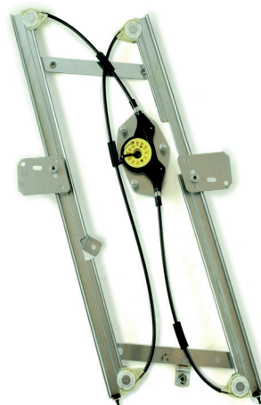
Our window regulator - notre lève-vitre - unser Fensterheber - nuestro eleva-lunas- nosso levantator de vidro - Γρύλος γνήσιος - nostro alzacristallo
