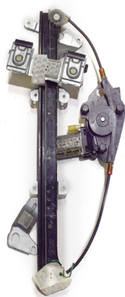
oem window regulator - lève-vitre original - Fensterheber von oem - elevalunas original - levantator de vidro original - Γρύλος γνήσιος - alzacrystallo originale
