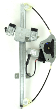
Our window regulator - notre lève-vitre - unser Fensterheber - nuestro elevalunas- nosso levantator de vidro - Γρύλος γνήσιος - nostro alzacrystallo
