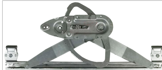
POWER WINDOW RIGHT ALZACRISTALLI ELETTRICO DX
