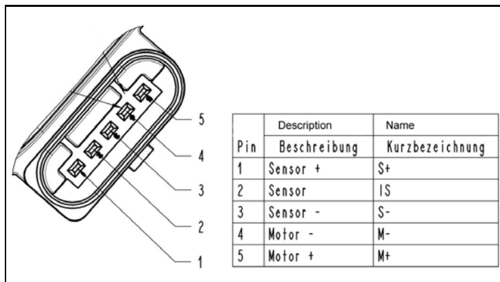
2 - Anschluss / Connector
