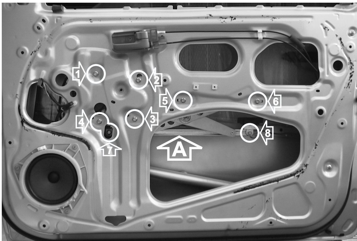
Porta lato destra - Right hand side door
