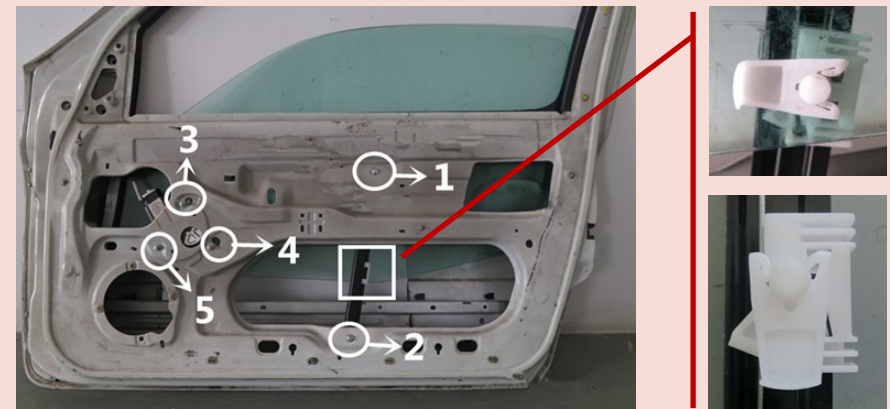
Vorne rechts/Front right (OE Ref. No. 7700 842 246)
