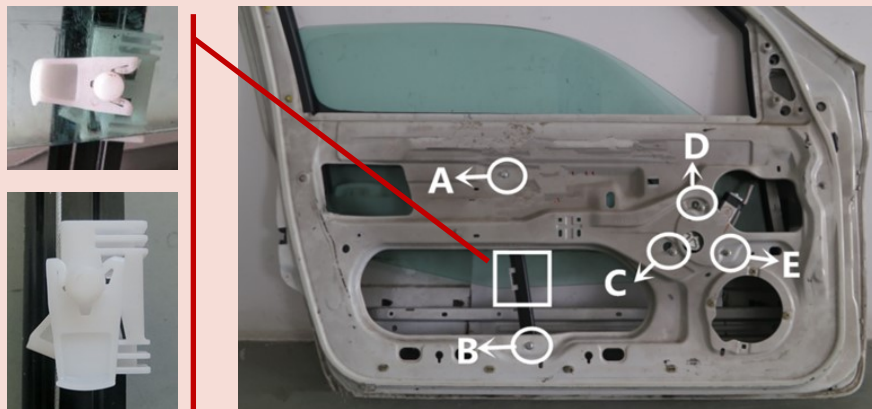
Vorne links/Front left (OE Ref. No. 7700 842 247)
