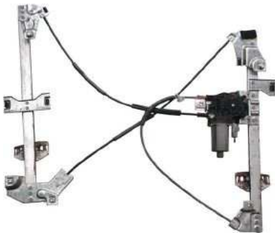
ALZACRISTALLO ELETTRICO ORIGINALE SINISTRO ORIGINAL POWER WINDOW LEFT
