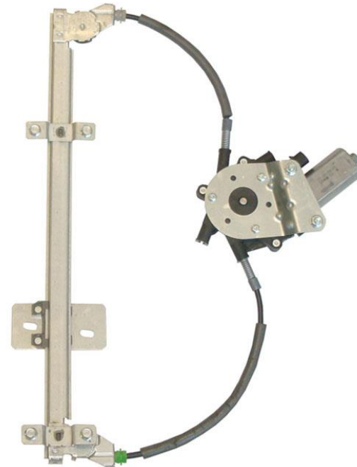
POWER WINDOW LEFT ALZACRISTALLI ELETTRICO SX
