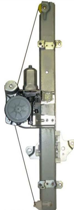
ORIGINAL POWER WINDOW RIGHT ALZACRISTALLI ELETTRICO ORIGINALE DX
