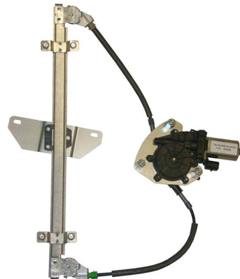
POWER WINDOW LEFT ALZACRISTALLI ELETTRICO SX
