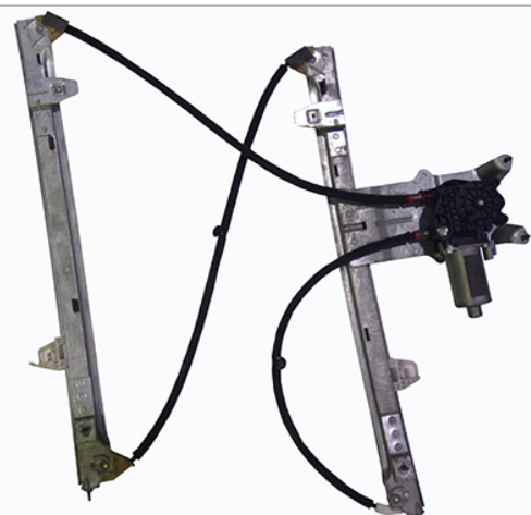
ORIGINAL POWER WINDOW ALZACRISTALLI ELETTRICO ORIGINALE
