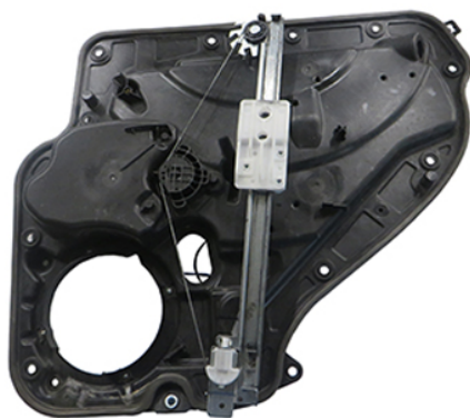
POWER WINDOW LIFTER ALZACRISTALLI ELETTRICO
