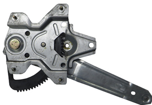
ORIGINAL POWER WINDOW RIGHT ALZACRISTALLI ORIGINALE ELETTRICO DX
