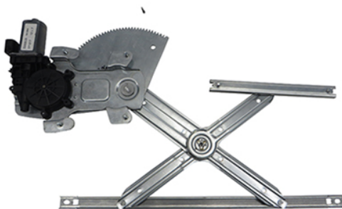
POWER WINDOW RIGHT ALZACRISTALLI ELETTRICO DX
