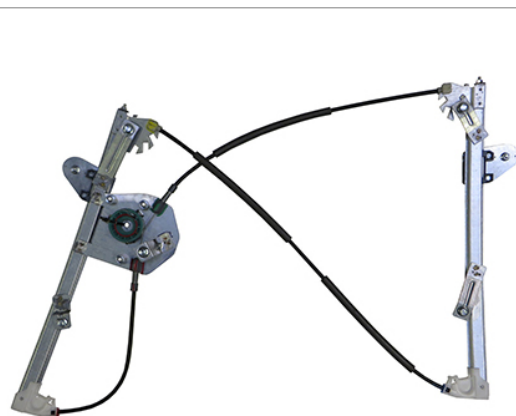
POWER WINDOW RIGHT ALZACRISTALLI ELETTRICO DX
