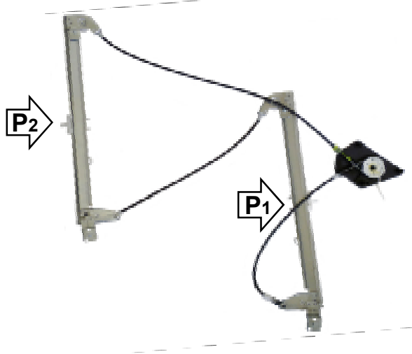
Ns meccanismo SX
