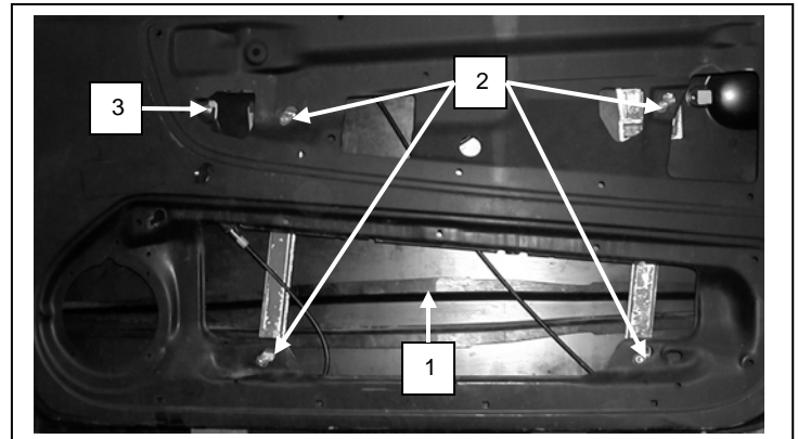
Puerta lado derecho, Right front door
