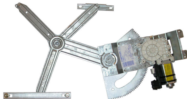
POWER WINDOW LEFT ALZACRISTALLI ELETTRICO SX
