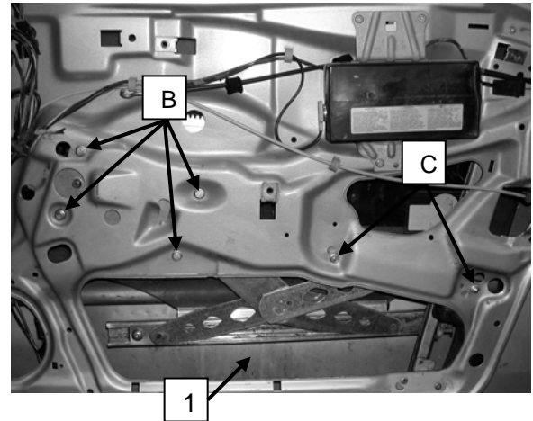
Puerta lado derecho, Right front door
