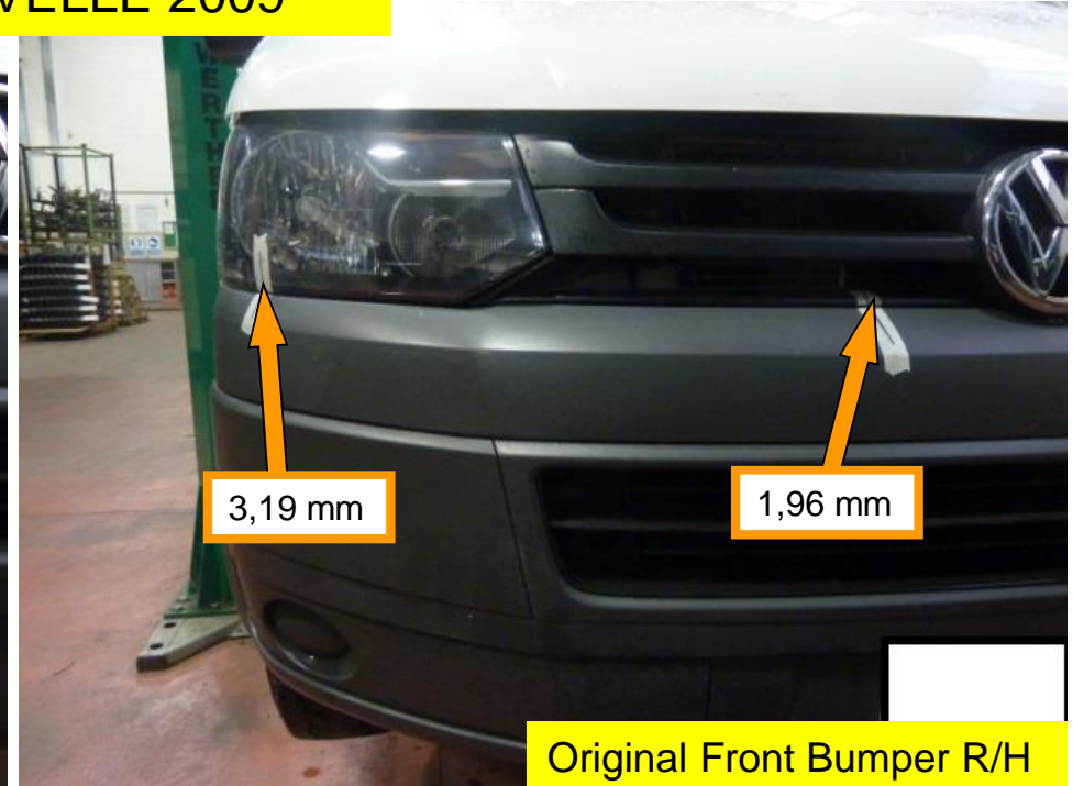
VW CARAVELLE 2009
