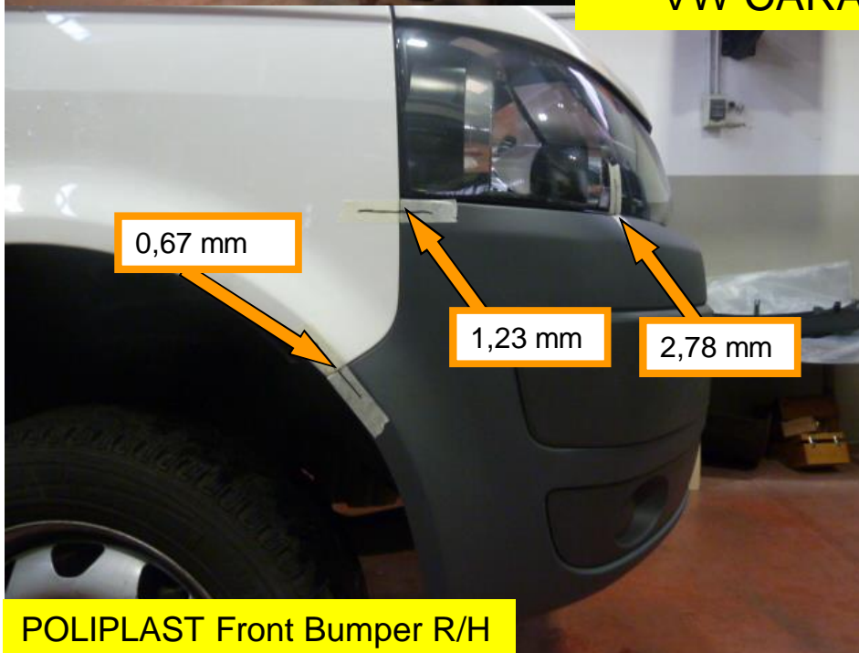
VW CARAVELLE 2009
