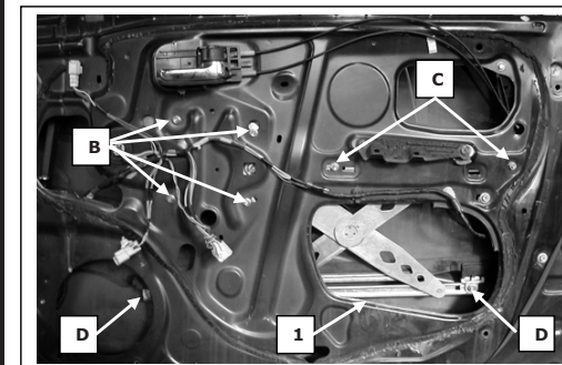
Porta lato destro, Portière avant droite, Right front door, Puerta lado derecho, Vorne rechte Tür, Porta frenté dirieta, Sag on kapi, νόρτα εμπρόσθια δεξιά
