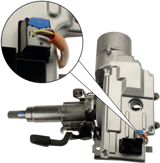
Harici sensör bağlantısına sahip direksiyon mili
