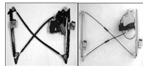
Alzacristallo originale - oem window regulator - lève-vitre original - Fensterheber von oem - elevalunas original - levandator de vidro original original cam acacagi - Γρύλος γνήσιος
