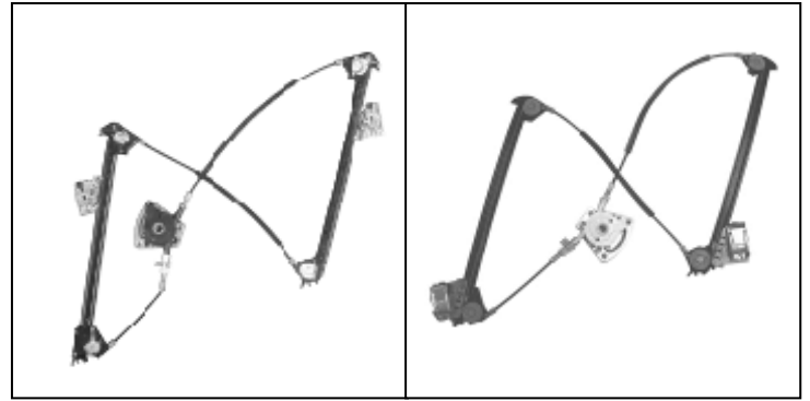
Elevavinas original – lève-vitre original – oem window regulator – levandator de vidro original Nuestro elevavinas – notre lève-vitre – our window regulator – nosso levantador de vidro
