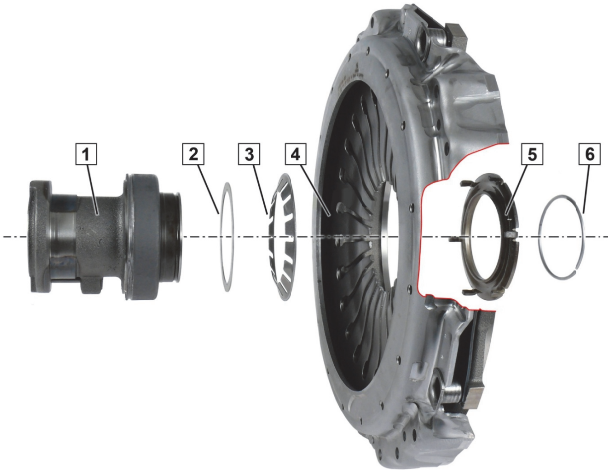
Abb. 1: Ausrücker mit Festverbindung. Montagereihenfolge und Ausrichtung der Bauteile
