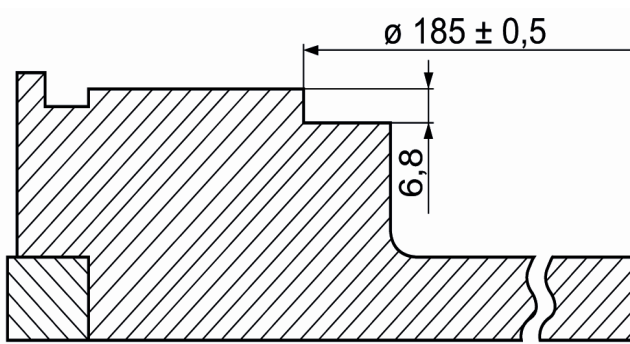
Fig. 1: Schwungrad / Flywheel / Volant moteur / Volante motor
