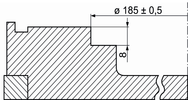
Fig. 2: Schwungrad nachgearbeitet / Refinished flywheel / Volant moteur après réfection / Volante motor rectificado
