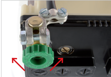
4. Schließen und Unterbrechen des Stromkreises
