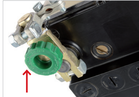
3. Montage der Quick Breaker-Klemme
