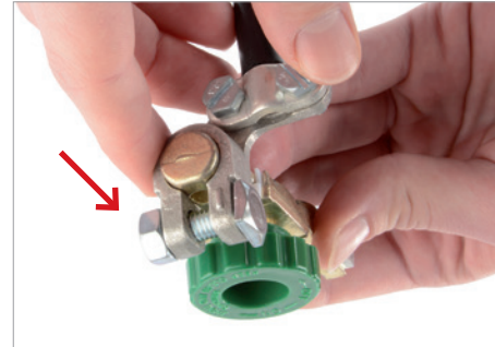
2. Montieren der Minusklemme an Quick Breaker-Klemme
